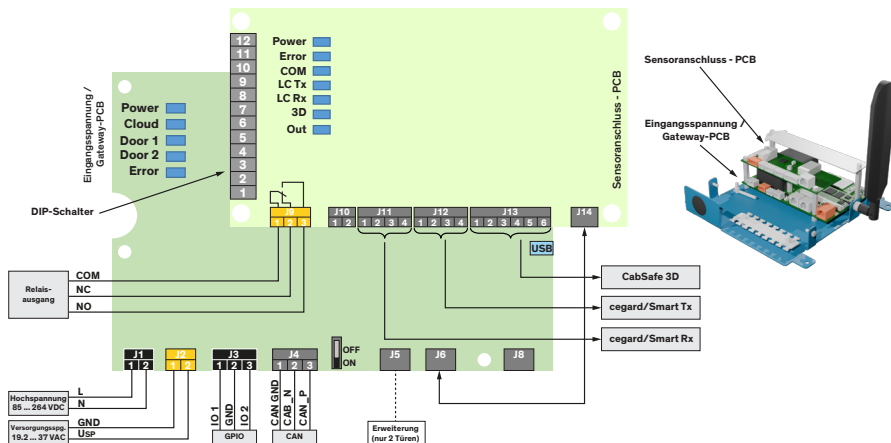
Abb 5: cegard/Smart PCB-Komponenten für ein cegard/Smart-Kontroller
