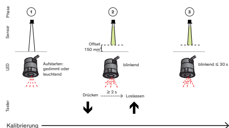
Abb 15: Konfiguration Typ T mit dem Teach-in-Taster
