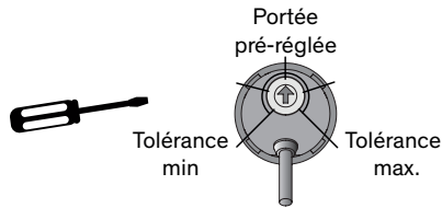
Figure 16 : Ajustement de la portée (+/-) selon le nom du capteur
