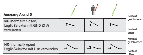
Abb 18: Logik-Selektor
