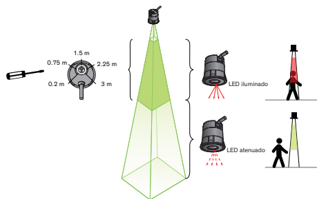
Figura 13: Configuración del tipo N
