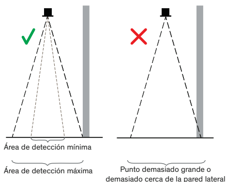
Figura 10: Amplitud de iluminación del TOF/Spot
