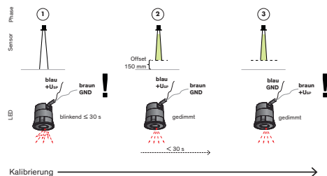
Abb 14: Konfiguration Typ T - Spannungswechsel
