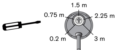
Abb 12: Beispiel für eine Einstellung zwischen 0.2 und 3 m
