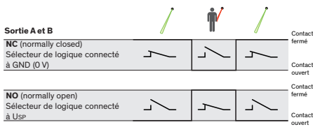
Figure 18 : Sélecteur de logique
