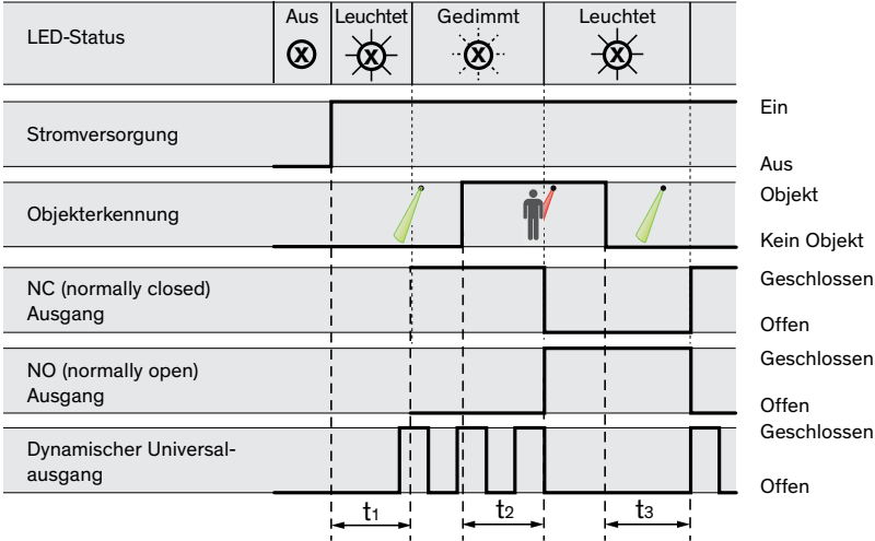
Abb 24: Zeitdiagramm - Relaisausgang
