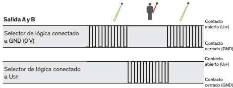
Figura 20: Selector de lógica, salida universal dinámica
