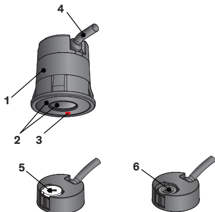
Abb 4: Übersicht TOF/Spot
